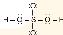
H 2 SO 4
