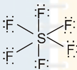
SF 6
